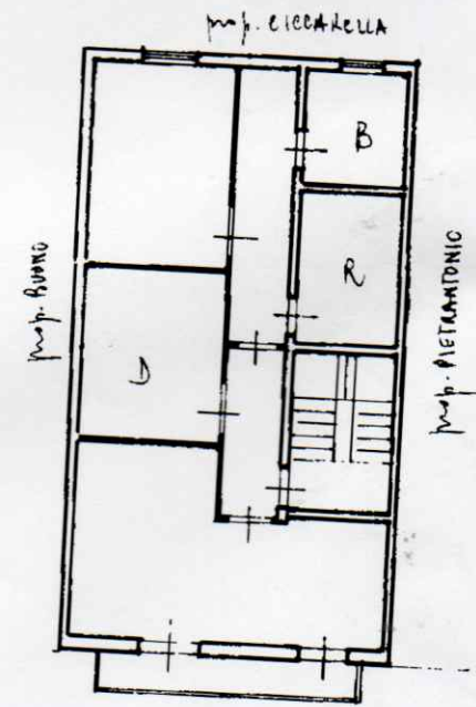
PIANTA PRIMO PIANO h=2.95
