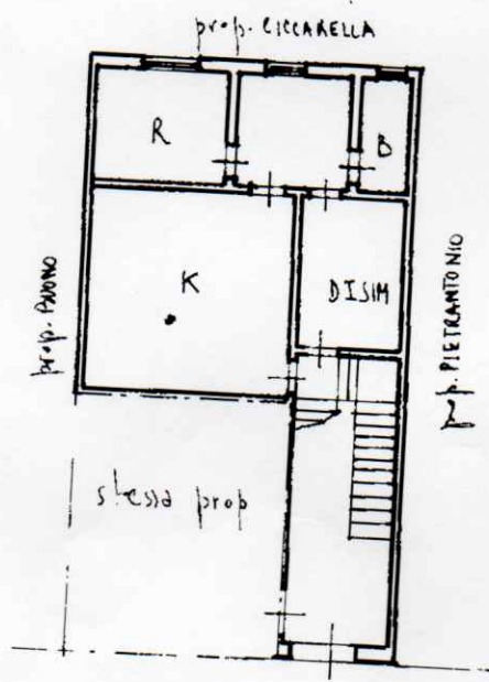
PIANTA PIANO TERRA h=3.55
